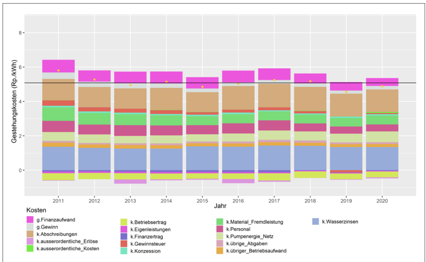
Bild 5: Spezifische Kosten (Rp./kWh) sämtlicher Kraftwerke für die Jahre 2011–2020 nach Kostenarten auf Stufe Kraftwerk. Gelbe Punkte: Gestehungskosten pro Jahr; schwarze Linie: durchschnittliche Gestehungskosten über alle Jahre und Kraftwerke. Abkürzungen: g.: «gemeinsame» Kostenarten auf Stufe Kraftwerk, die mit den kalkulatorischen Kapitalkosten auf Stufe Aktionär verrechnet werden ( siehe Bild 6 ); k.: Kostenarten auf Stufe Kraftwerk.
