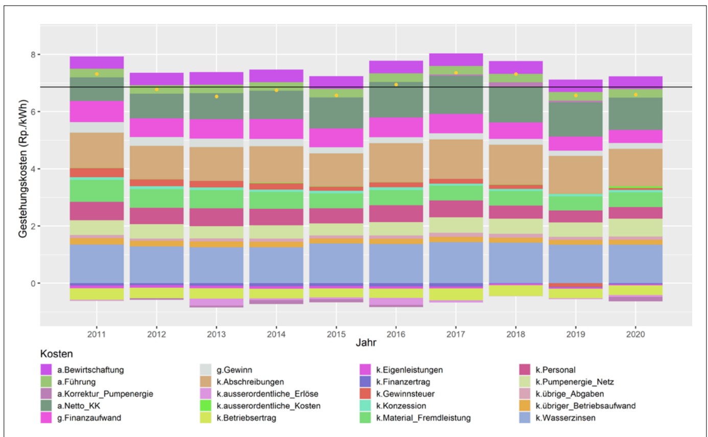
Bild 7: Spezifische Kosten (Rp./kWh) sämtlicher Kraftwerke für die Jahre 2011–2020 nach Kostenarten auf Stufe Betreiber. Gelbe Punkte: Gestehungskosten pro Jahr; schwarze Linie: durchschnittliche Gestehungskosten über alle Jahre und Kraftwerke.
